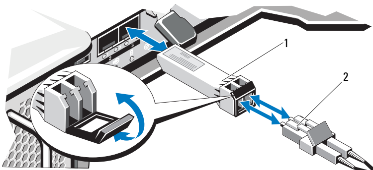
图 3-2. 光纤电缆连接
